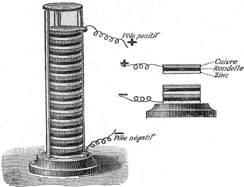
La pile de Volta (1800) composée d'un empilement de disque de zinc et de cuivre séparé par un feutre imprégné d'eau salée
