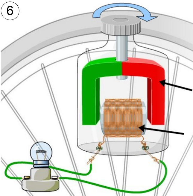
Alternateur simple
