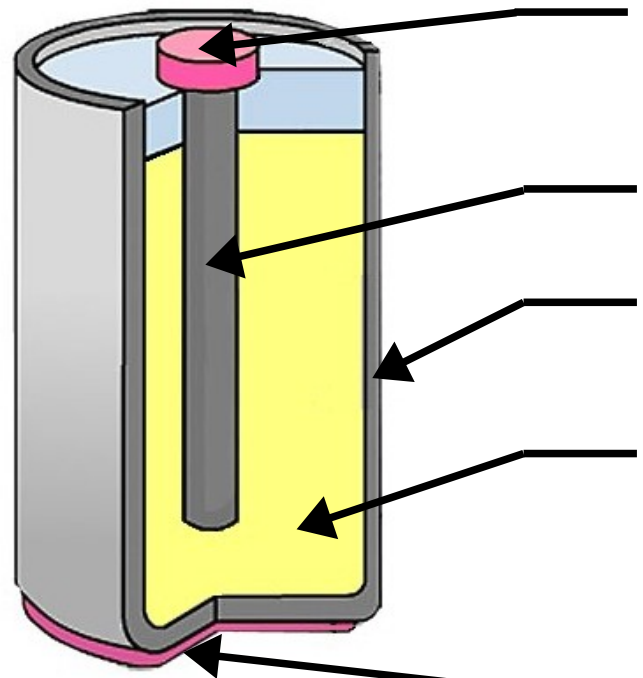
La pile Leclanché (1867) au zinc/charbon est très utilisée
